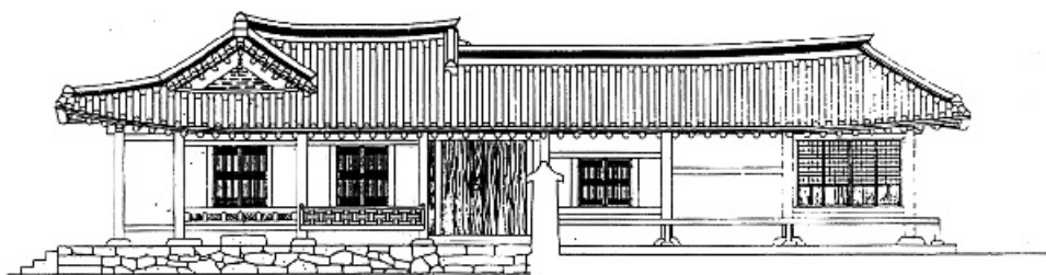
영암댁 사랑채 측면도
