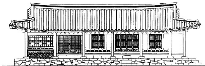
영암댁 사랑채 정면도
