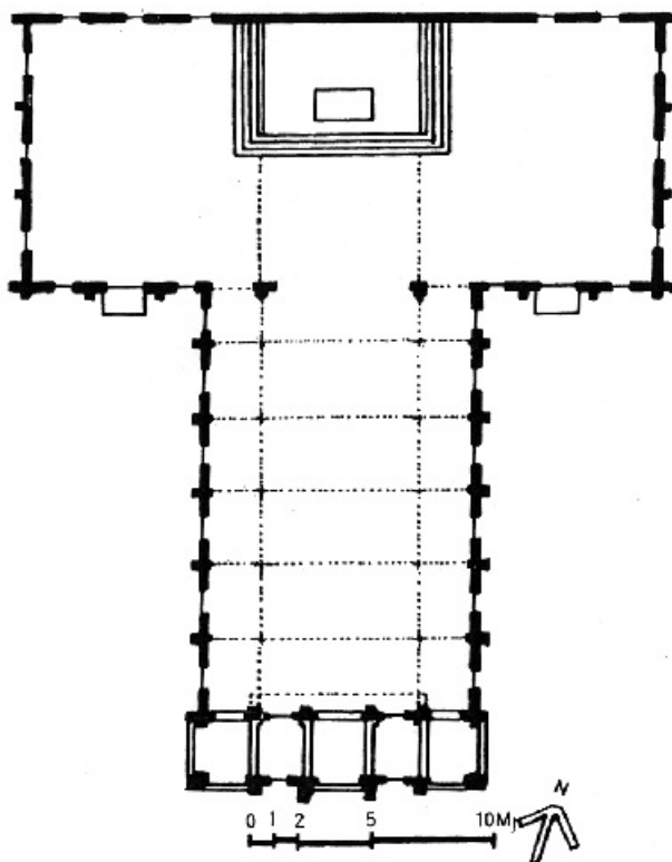
「공세리 천주교 성당 평면도」
